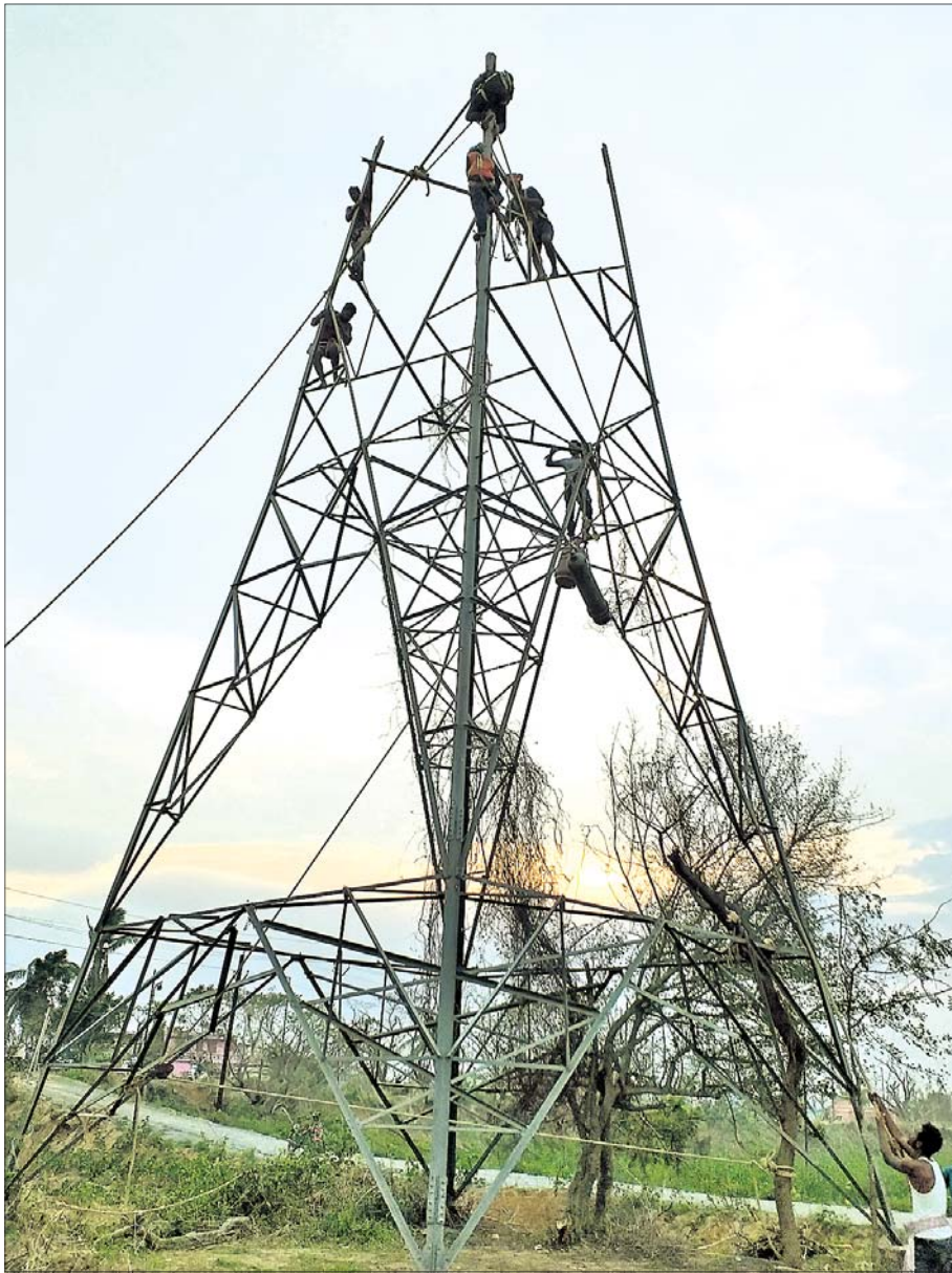
ବାଟ୍ୟା ‘ଫନ’ ପ୍ରକାଶରେ ପାଣ୍ଡରା ରୋଡ୍ ନିକଟରେ ଭାଙ୍ଗି ପଡ଼ିଥିବା ବିଦ୍ୟୁତ୍ ଟାଓରର ମରାମତି କାର୍ଯ୍ୟ ଚାଲିଛି।
