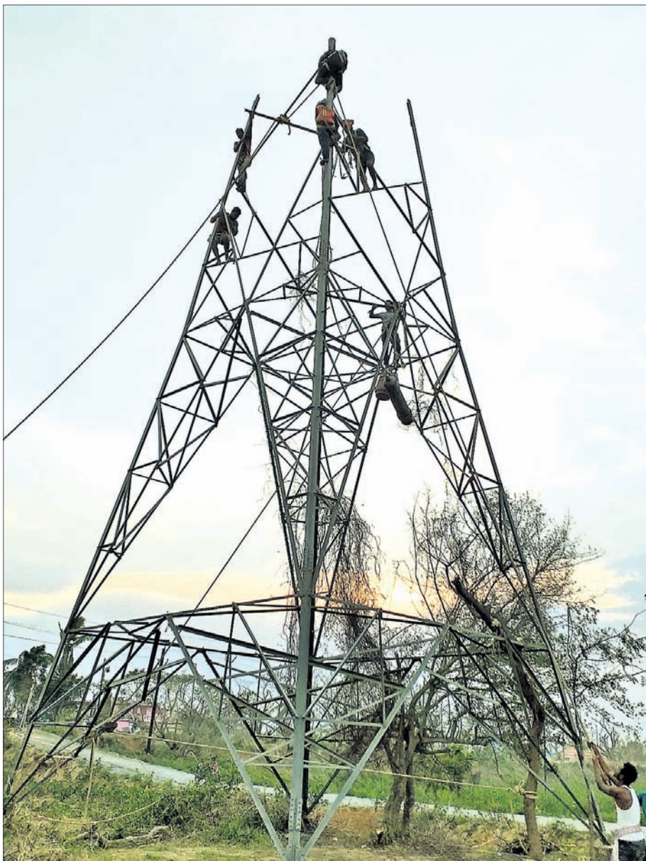
ଫନୀ ପ୍ରଭାବରେ ଭୁବନେଶ୍ୱର ଉପକଣ୍ଠ ପାଖରା ରୋଡ଼ ନିକଟରେ ଭାଙ୍ଗି ପଡ଼ିଥିବା ବିଦ୍ୟୁତ୍ ଟାଓ୍ୱାରର ମରାମତି କାର୍ଯ୍ୟ ଚାଲିଛି।
