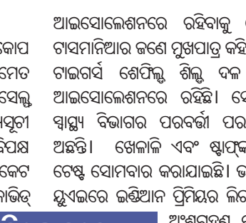
ପେନ୍ ସିଦ୍ଧାନ୍ତ
