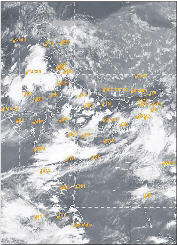
ଶୁକ୍ରବାର ଅପରାହ୍ନ ୫ଟାରେ ମହାକାଶରୁ ଉଦ୍ଧୋଳିତ ପାଣିପାଗର ଚିତ୍ର ।
